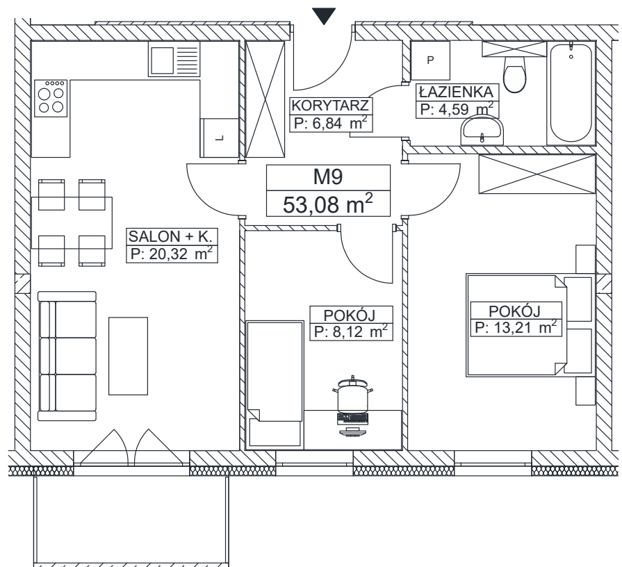
Rzut lokalu
