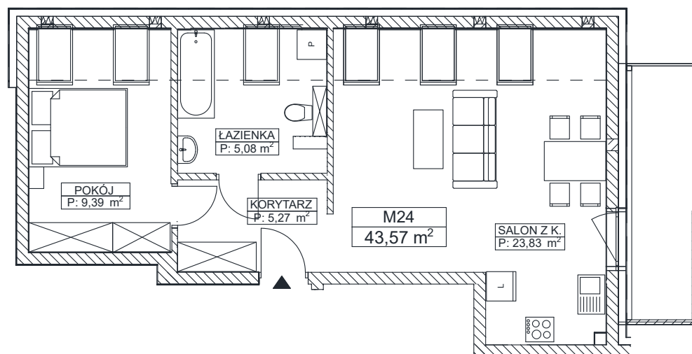
Rzut lokalu
