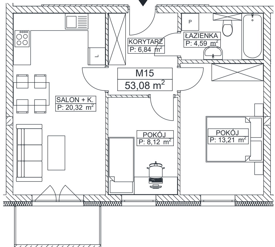
Rzut lokalu
