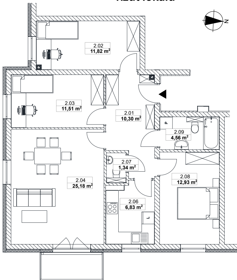
Rzut lokalu
