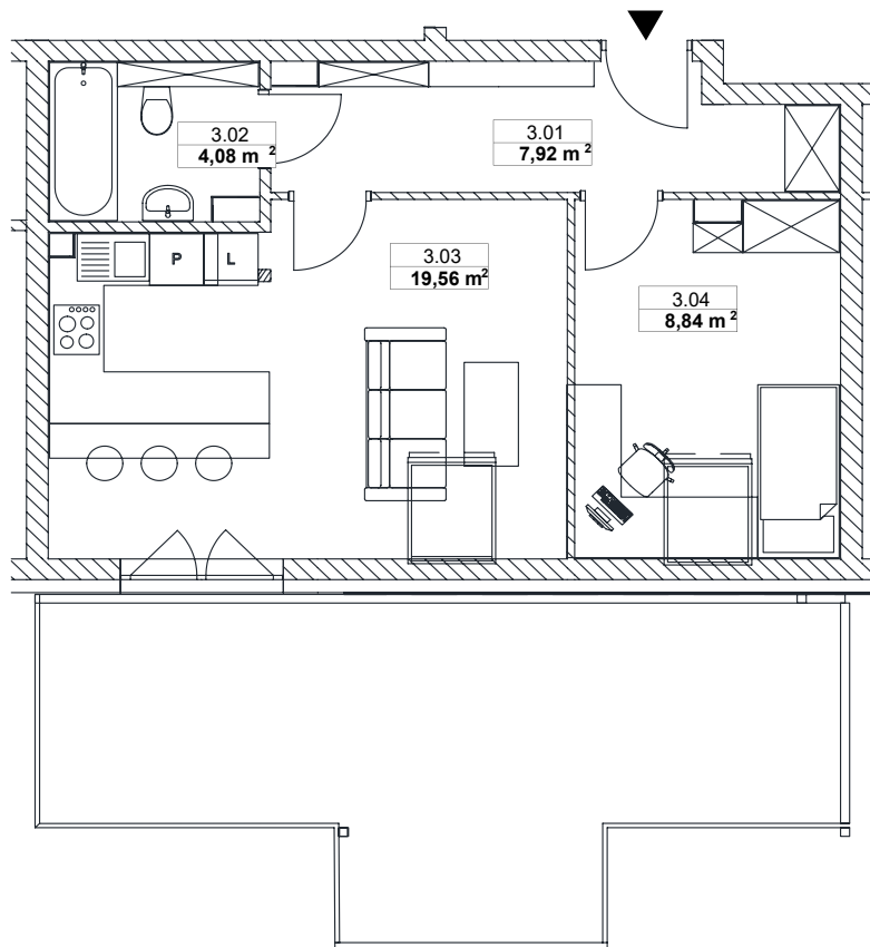
Położenie lokalu na rzucie kondygnacji
