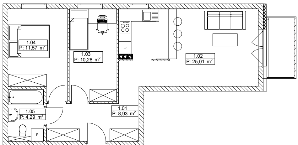
Rzut lokalu
