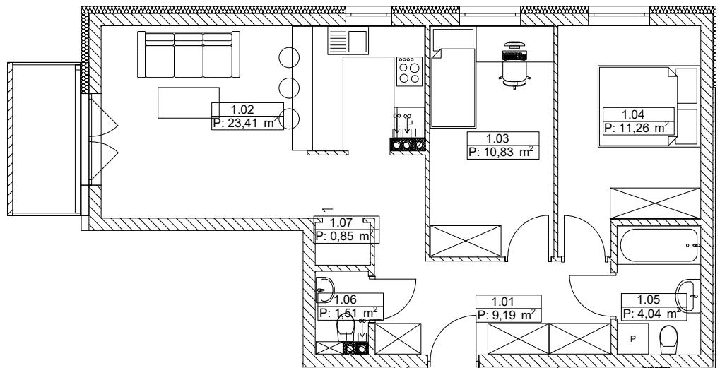
Rzut lokalu
