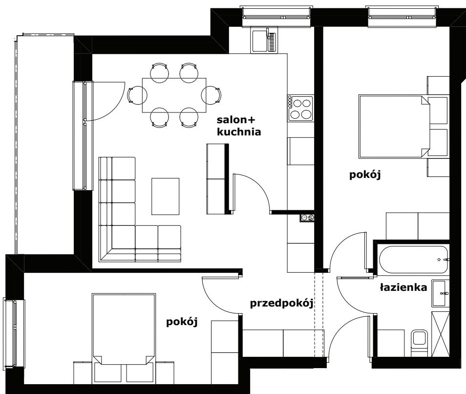
Rzut lokalu
