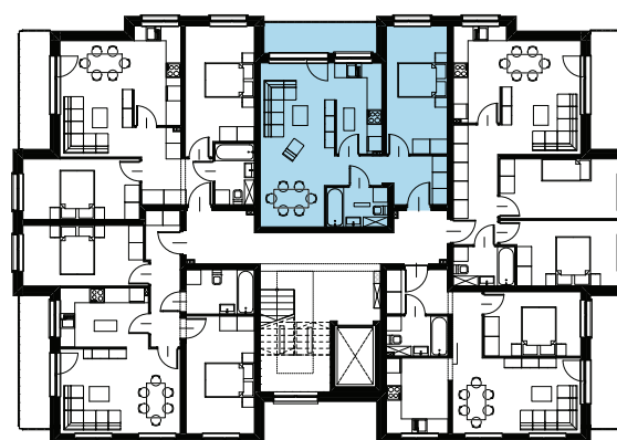
Położenie lokalu na rzucie kondygnacji
